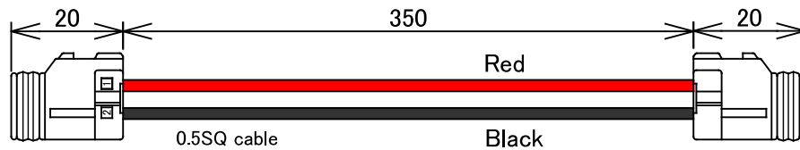
WCSHL-2RC (2 pin)
