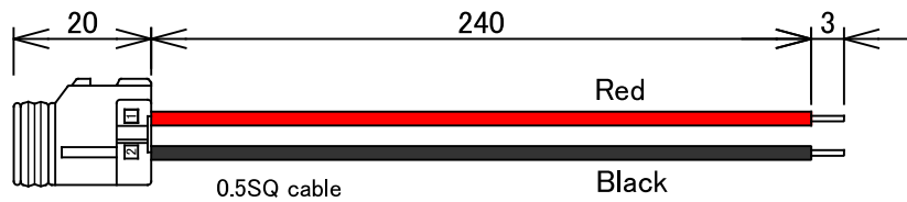
WCSHL-2PC (2 pin)
