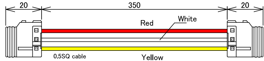
WCSHL-3RC (3 pin)
