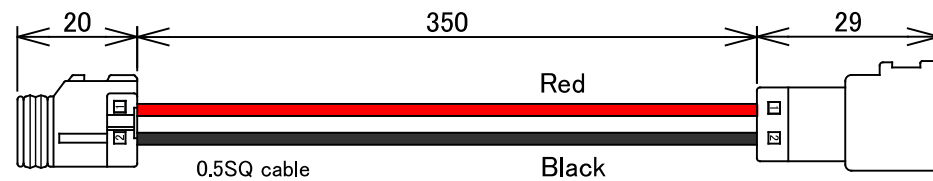
WCSHL-2TC (2 pin)
